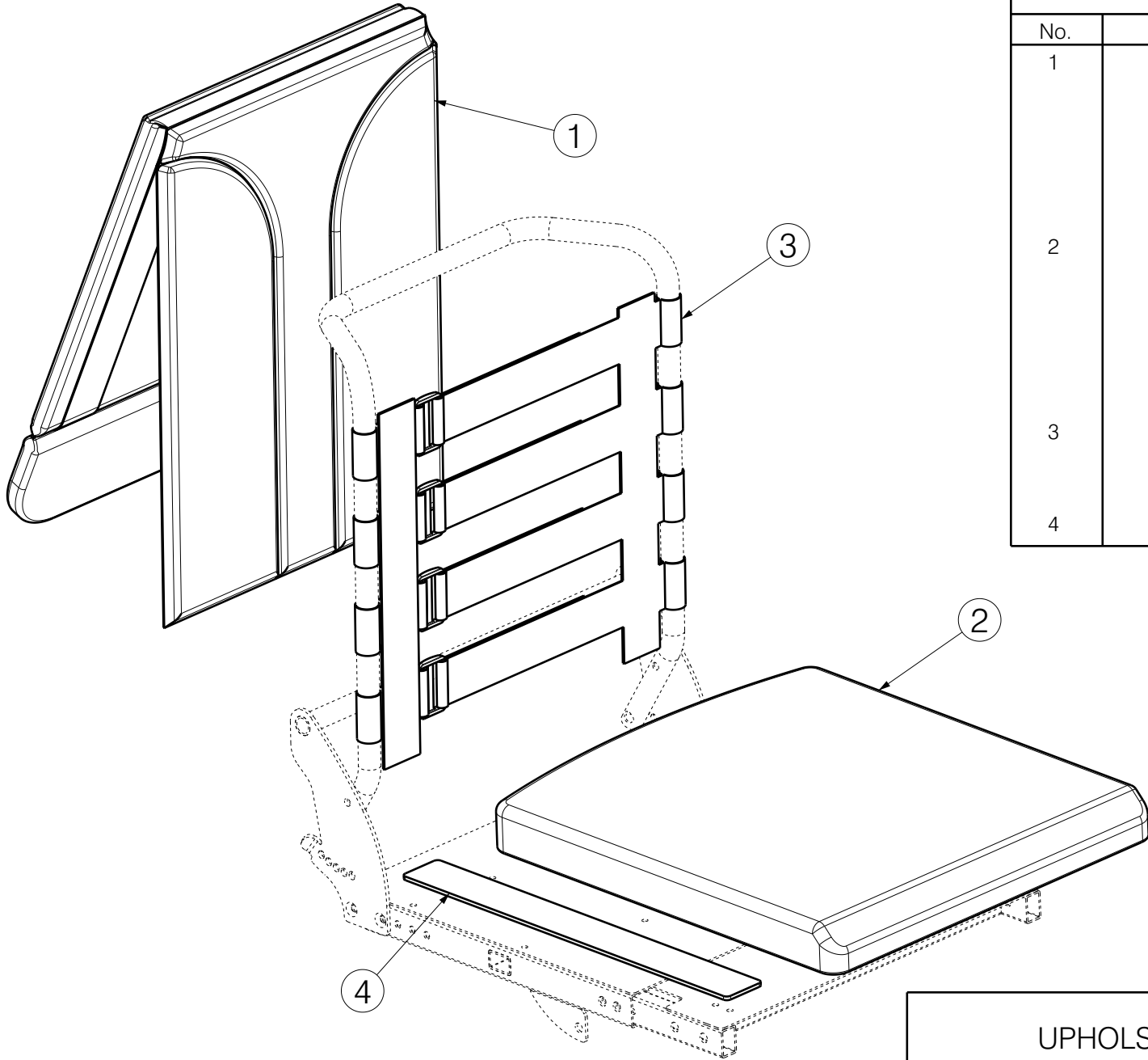
Isometric view Scale: 1:6
